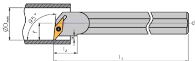
Utensile per tornitura interna A.. SVLC R/L TA6114, con stelo in acciaio.
