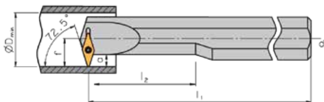
Utensile per tornitura interna A.. SVVC R/L TA6117, con stelo in acciaio.
